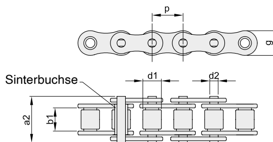
Sinterbuchsen
