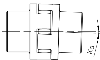
Winkerversatz
