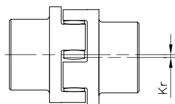
Radialversatz
